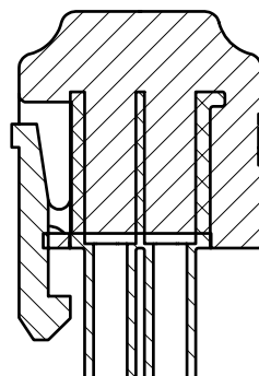
A-A ( 2,50 : 1 )
